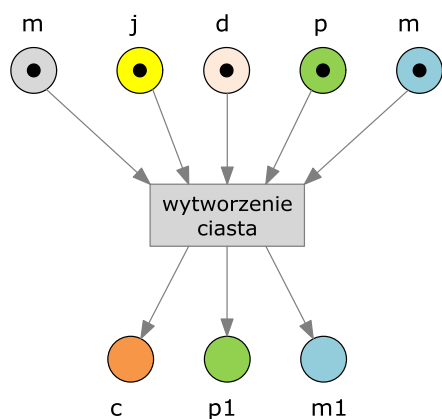
Rys.2.1 Tranzyt przed odpaleniem
