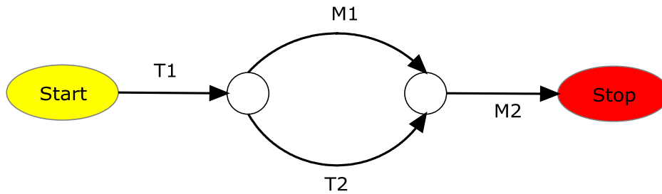
Rys.5.1 Tynkowanie i malowanie opisane siecią PERT
