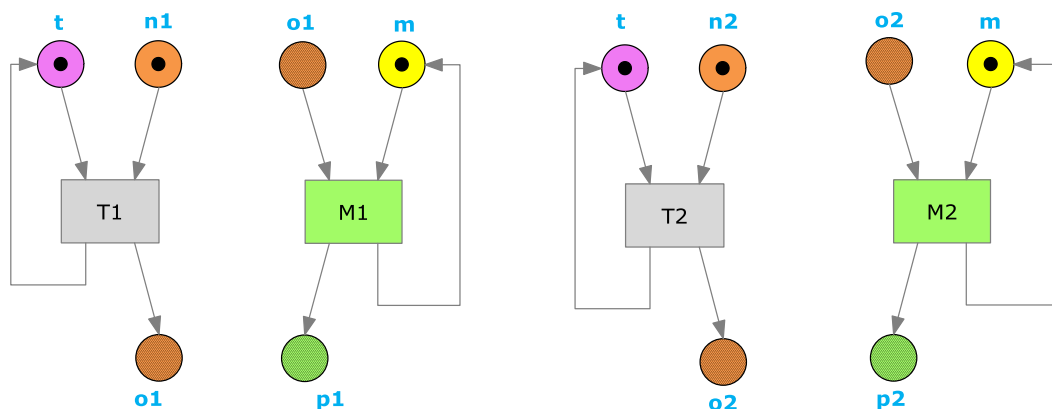
Rys. 3.1 Cztery atomy
