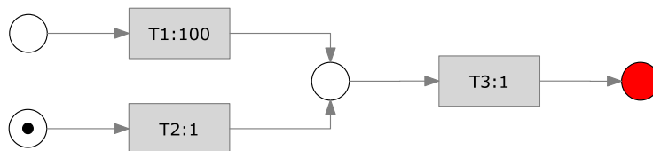
Rys.14.1 Sieć z martwym tranzytem
